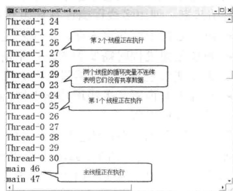
图 16.1 多线程运行的效果
