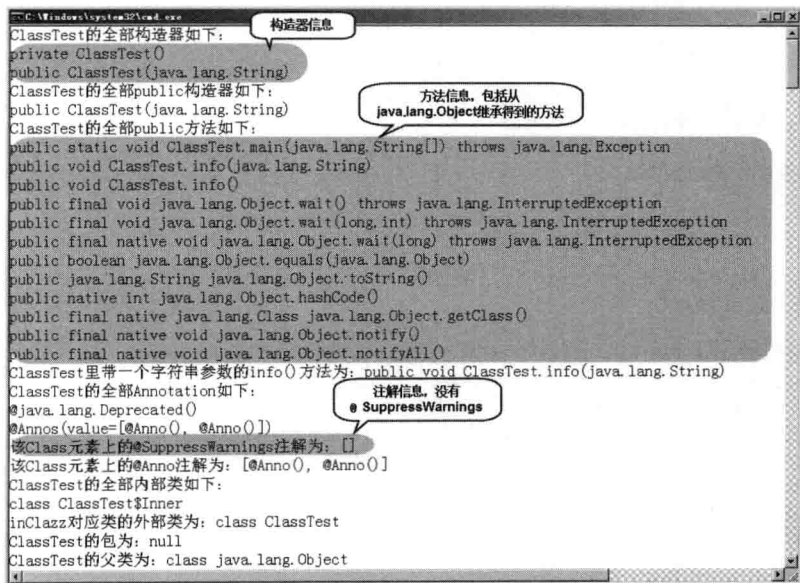
图 18.2 使用 Class 对象查看该类的内部信息
