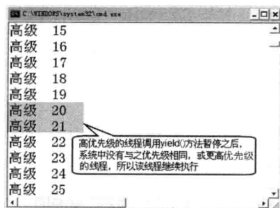
图 16.7 线程调用 yield()方法暂停后再次被调度执行
