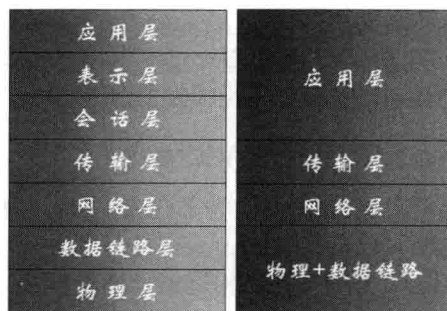
图 17.2 OSI 分层模型和 TCP/IP 分层模型的对应关系
