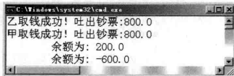
图 16.9 线程同步的问题
