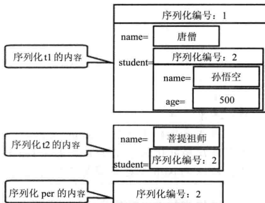
图 15.14 序列化机制示意图
