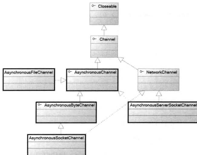
图 17.7 AIO 的接口和实现类
