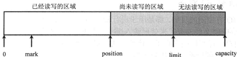
图 15.16 Buffer 读入数据后的示意图
