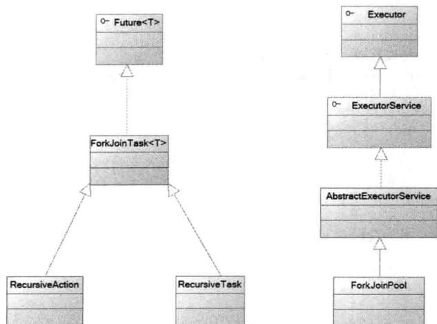
图 16.16 线程池工具类的类图
