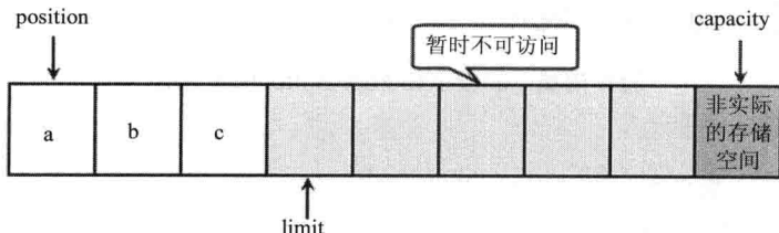
图 15.19 执行 Buffer 的 flip() 方法后的示意图
