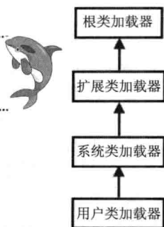
图 18.1 JVM 中 4 种类加载器的层次结构
