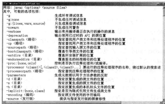
图 15.12 Java 程序获得 javac 命令的错误输出
