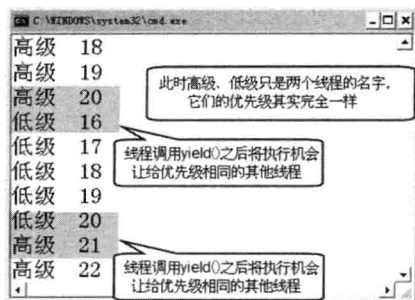
图 16.6 线程调用 yield()方法后将执行机会让给优先级相同的其他线程
