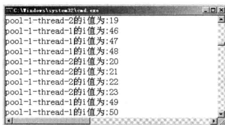
图 16.15 使用线程池并发执行两个任务
