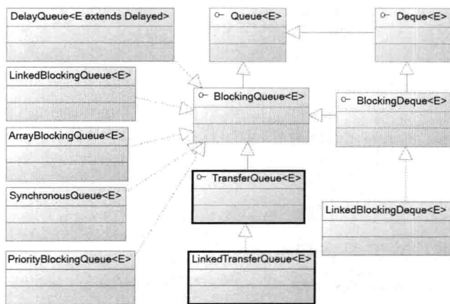
图 16.13 BlockingQueue 与其实现类之间的类图
