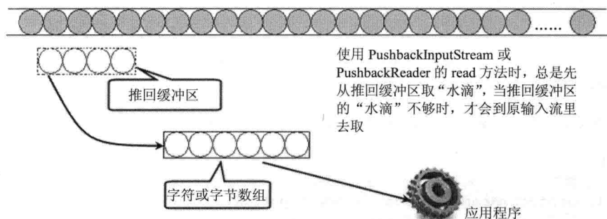
图 15.10 推回输入流的处理示意图
