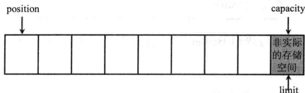
图 15.17 新分配的 CharBuffer 对象
