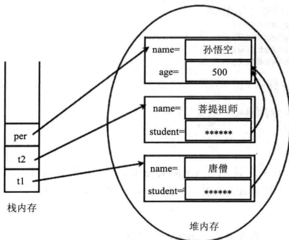
图 15.13 两个 Teacher 对象的 Student 实例变量都引用到同一个 Person 对象
