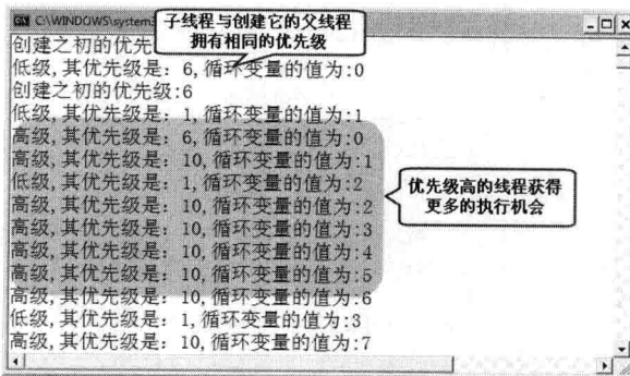
图 16.8 改变线程优先级的效果
