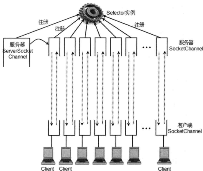
图 17.6 NIO 的非阻塞式服务器示意图
