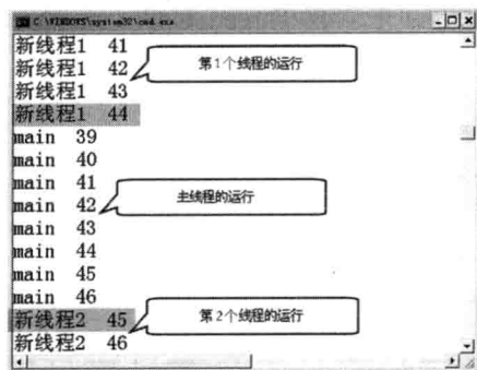
图 16.2 实现 Runnable 接口创建的多线程
