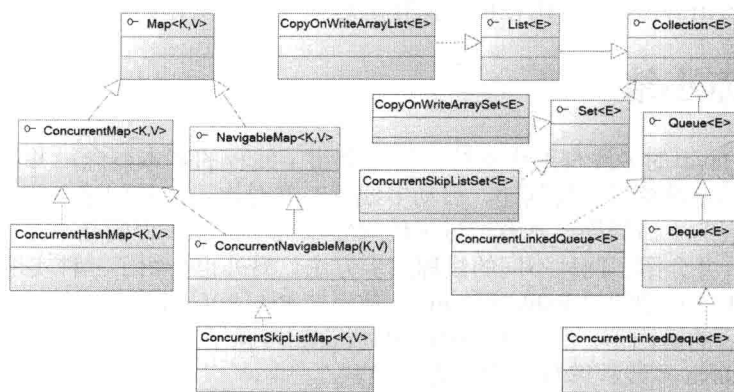
图 16.19 线程安全的集合类
