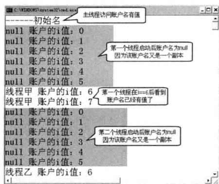
图 16.18 线程局部变量互不干扰的情形
