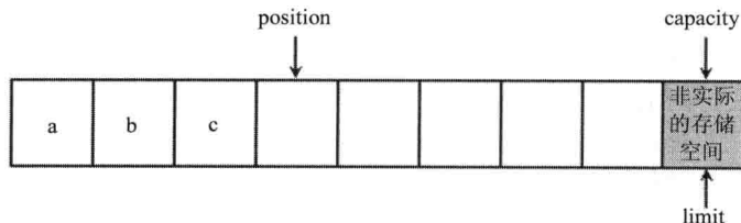
图 15.18 向 Buffer 中放入 3 个对象后的示意图
