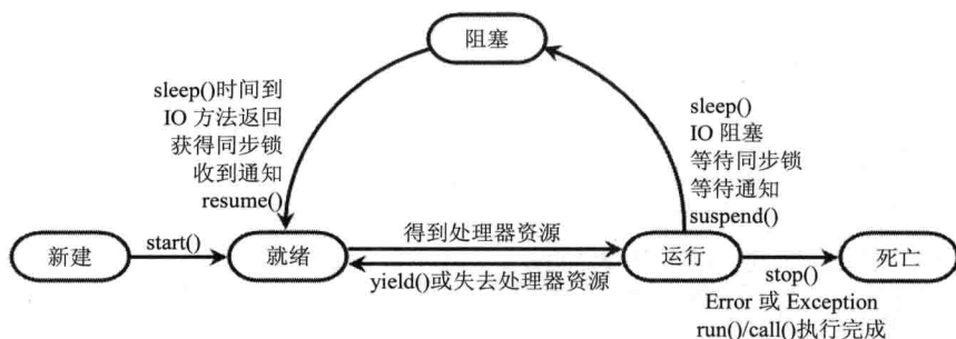
图 16.4 线程状态转换图
