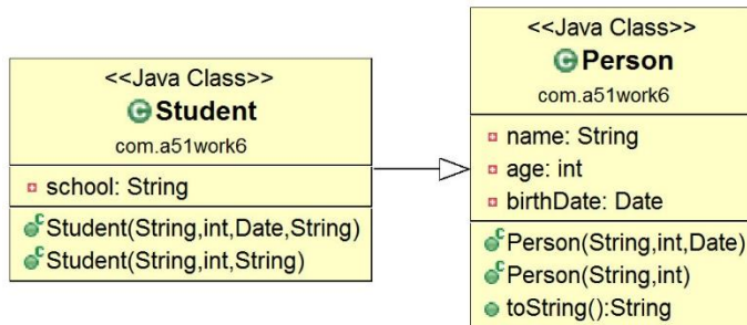
图 12-4 Person 和 Student 类图
