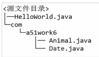
图 10-2 文件系统目录与包
