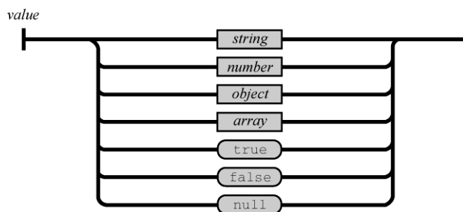
图 17-7 JSON 值的语法结构图
